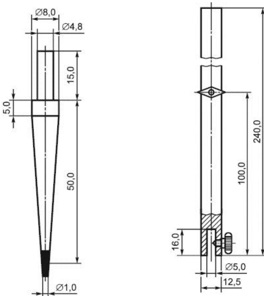
а) Съемный конус, материал - сталь
