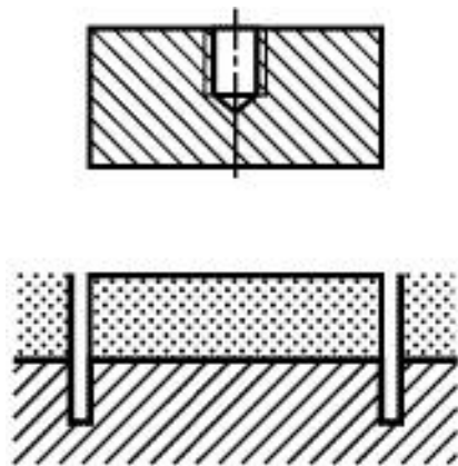
Рисунок 9 - Разрушение по слою клея (испытание следует повторить)
