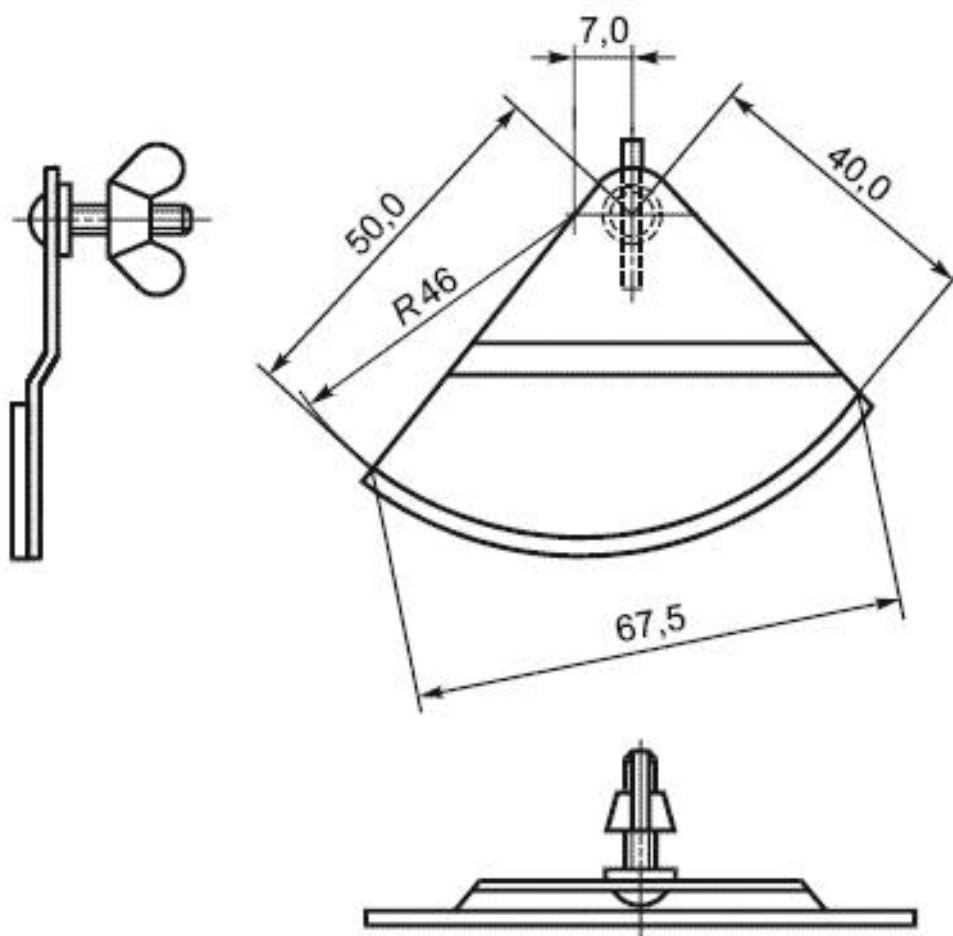
Рисунок 2 - Пластинка-фиксатор подвижного стержня с конусом
