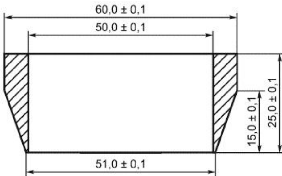
Рисунок 5 - Усеченное коническое кольцо
