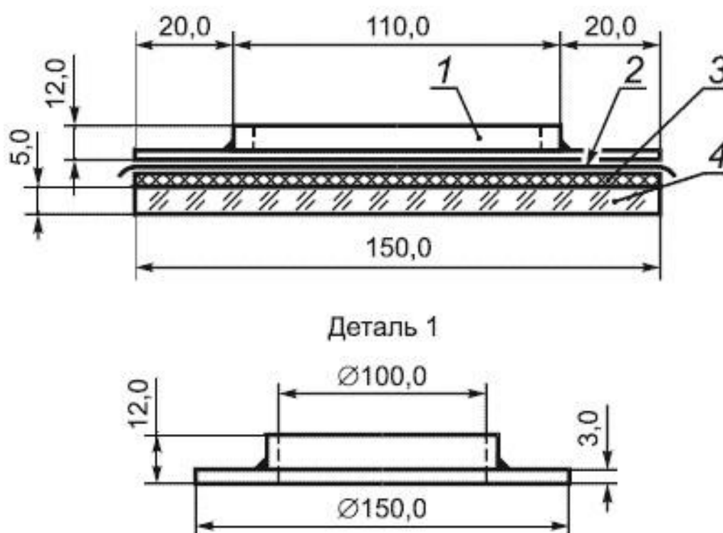
Рисунок 4 - Схема устройства для определения водоудерживающей способности
